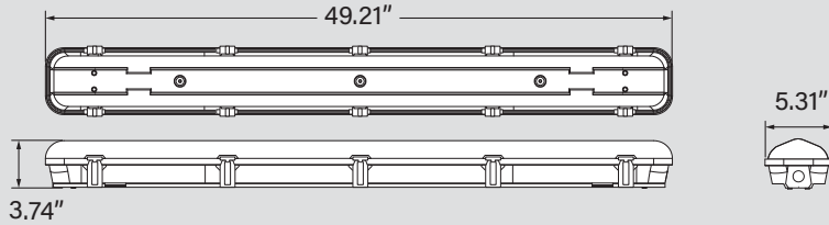
KT-VTLED75PS-M4A-8CSA-VDIM
