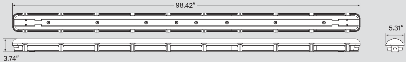
KT-VTLED100PS-M8A-8CSA-VDIM
